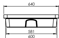
PE Verstärkung
