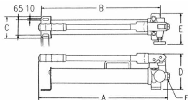
Combi-Satz PB 700
