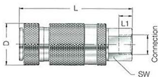
Innengewinde
