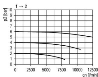
Durchflussdiagramm
