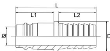
Einstecktülle
