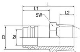
Nippel Außengewinde
