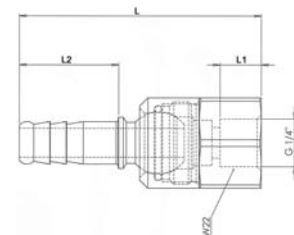
Schlauchtülle, Innengewinde
