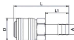
Schlauchtülle
