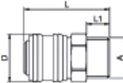
Außengewinde
