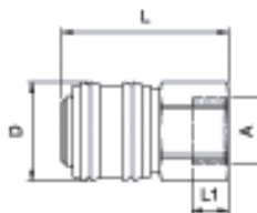
Innengewinde
