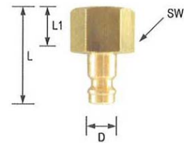
Nippel Innengewinde
