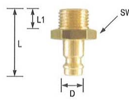
Nippel Außengewinde
