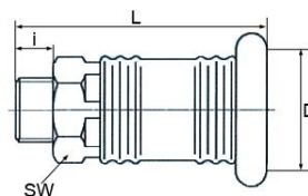
Außengewinde
