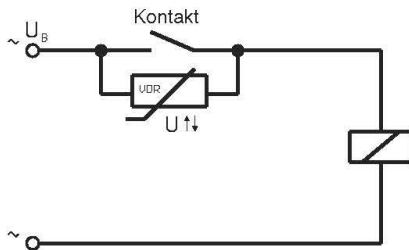
Beispiel: Kontaktschutzmaßnahme mit spannungsabhängigem Widerstand VDR
