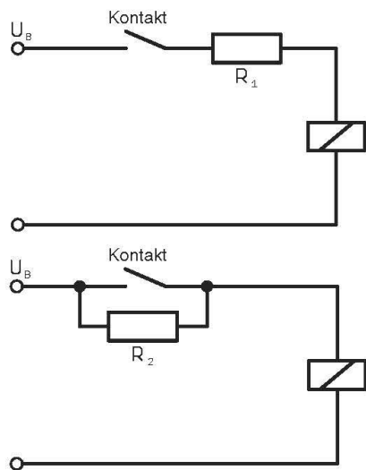
Beispiel: Kontaktschutzmaßnahme mit Widerstand zur Strombegrenzung
