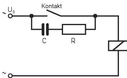
Beispiel: Kontaktschutzmaßnahme mit RC-Glied
