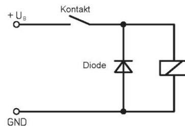
Beispiel: Kontaktschutzmaßnahme mit Freilaufdiode
