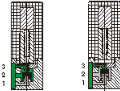
Stellung 1 (Ruhestellung)
